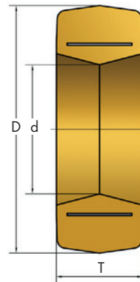
konischer Reifenfuß mittengeteilt (symmetrisch)
